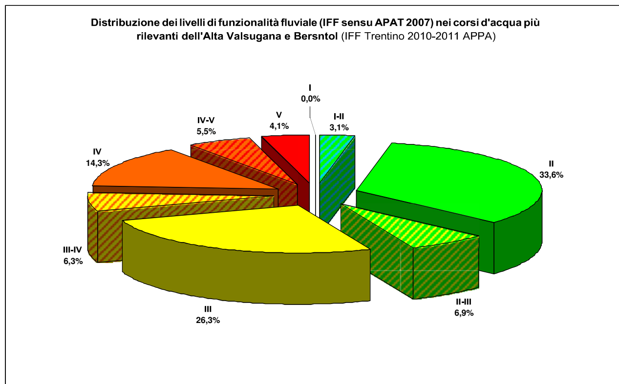
Fig. 3 - Rappresentazione grafica della distribuzione relativa dei livelli di Funzionalità Fluviale in Alta Valsugana (fonte: Progetto IFF Trentino2010-2011 - APPA).
